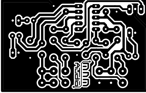
BOT & MASK 63 90mm x 40 00mm
