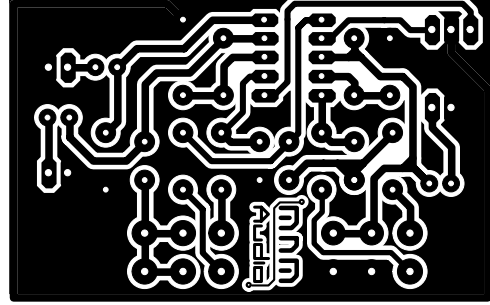
BOT & MASK 63 90mm x 40 00mm
