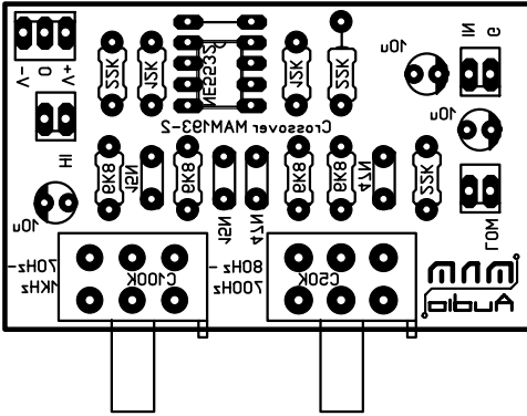
BOT & MASK 63 90mm x 40 00mm
